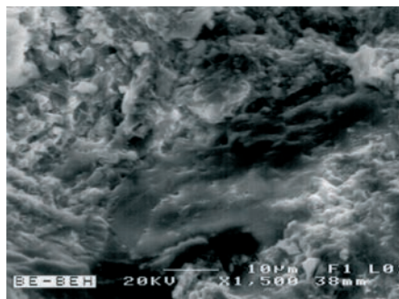
Abb. 8: Elektronenstrahlmikroskopische Aufnahmen von Betonboden-Oberflächen: links unbehandelt, Mitte und rechts behandelt (links und Mitte 1.500-fach vergrößert, rechts 4.000-fach vergrößert).
