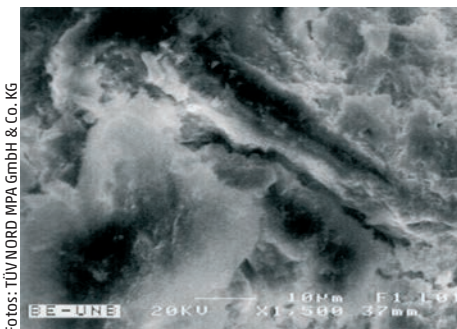
Abb. 8: Elektronenstrahlmikroskopische Aufnahmen von Betonboden-Oberflächen: links unbehandelt, Mitte und rechts behandelt (links und Mitte 1.500-fach vergrößert, rechts 4.000-fach vergrößert).
